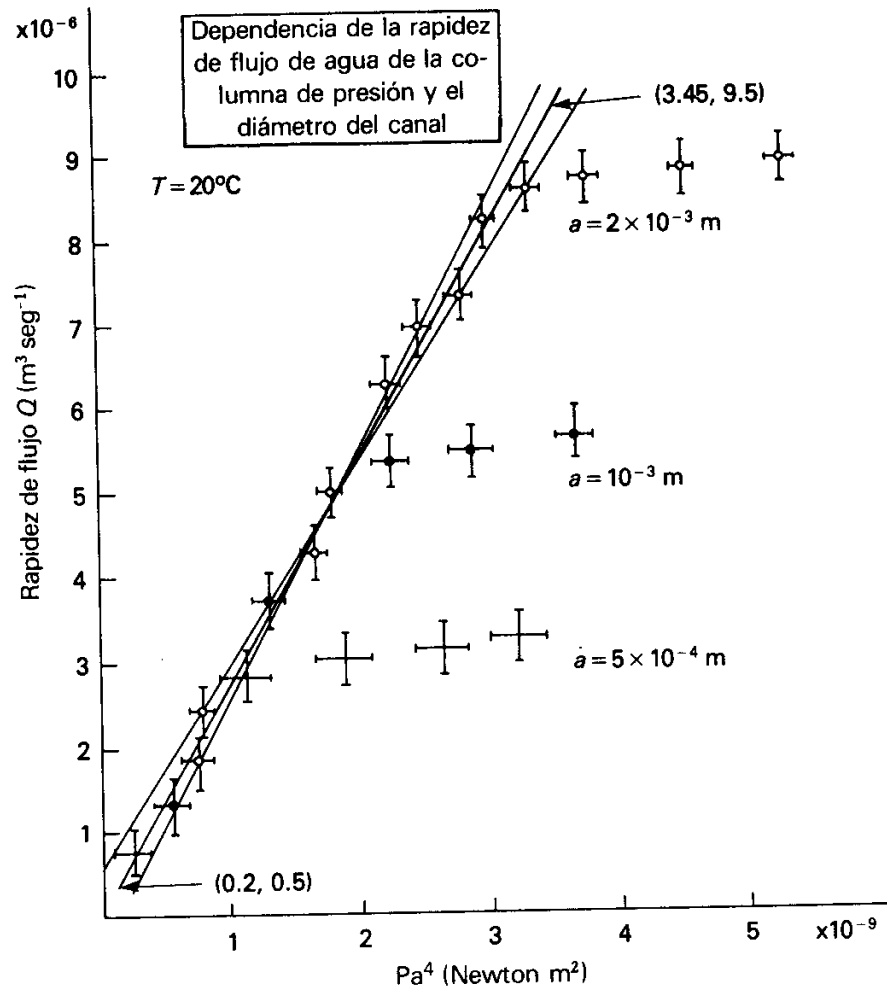
Figura 7-2 Una gráfica completa.
