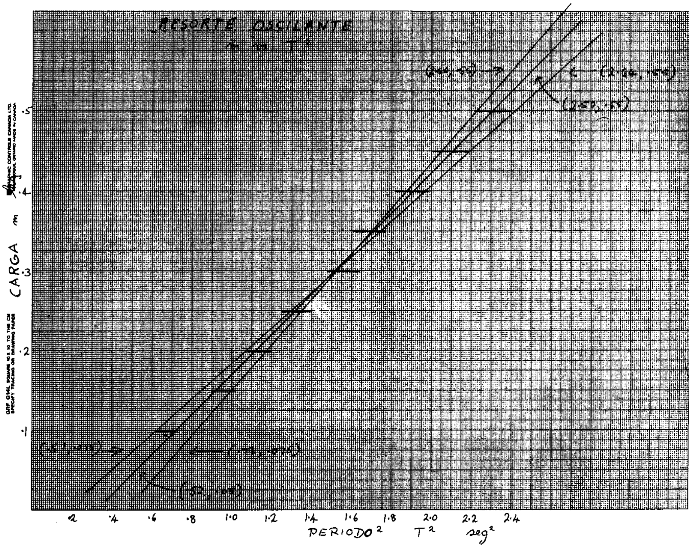
Figura A4-2 Forma final de la gráfica de m vs. T^2 .
