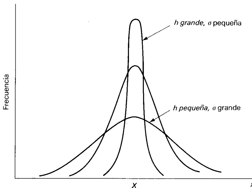
Figura 3-3 La curva de distribución Gaussiana.
