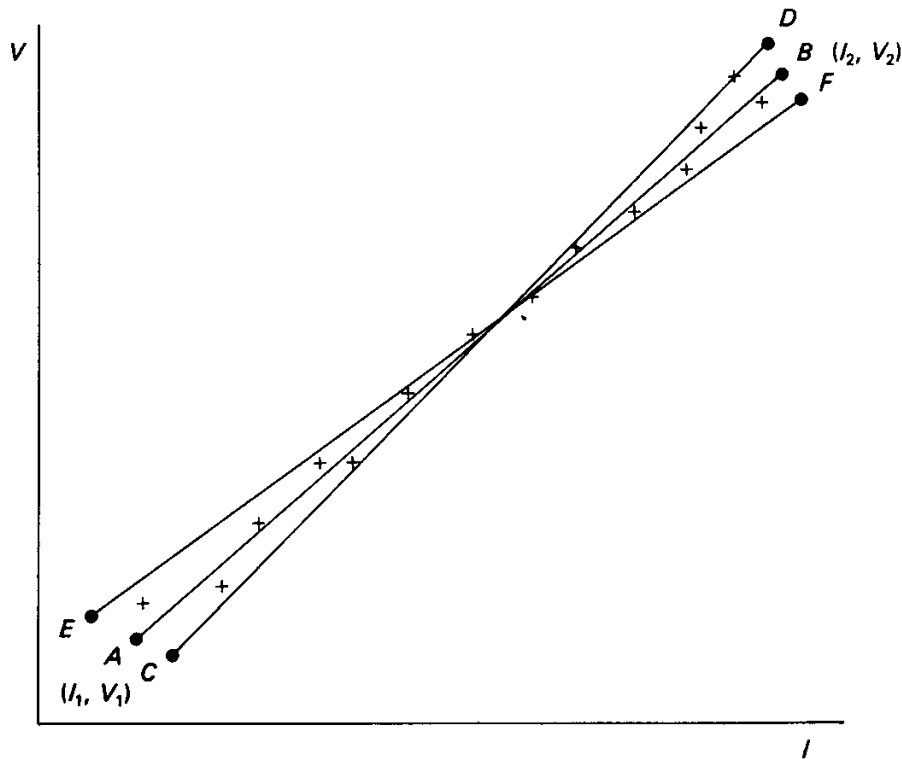
Figura 6-3 La “mejor” pendiente y sus límites extremos.
