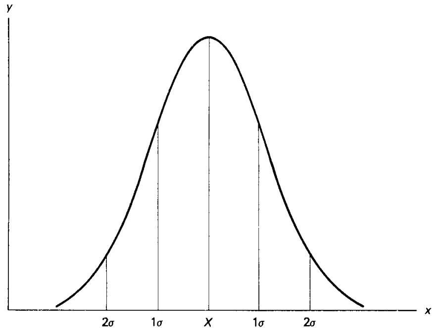
Figura 3-4 La relación de 1\sigma y 2\sigma con los límites de la distribución Gaussiana.
