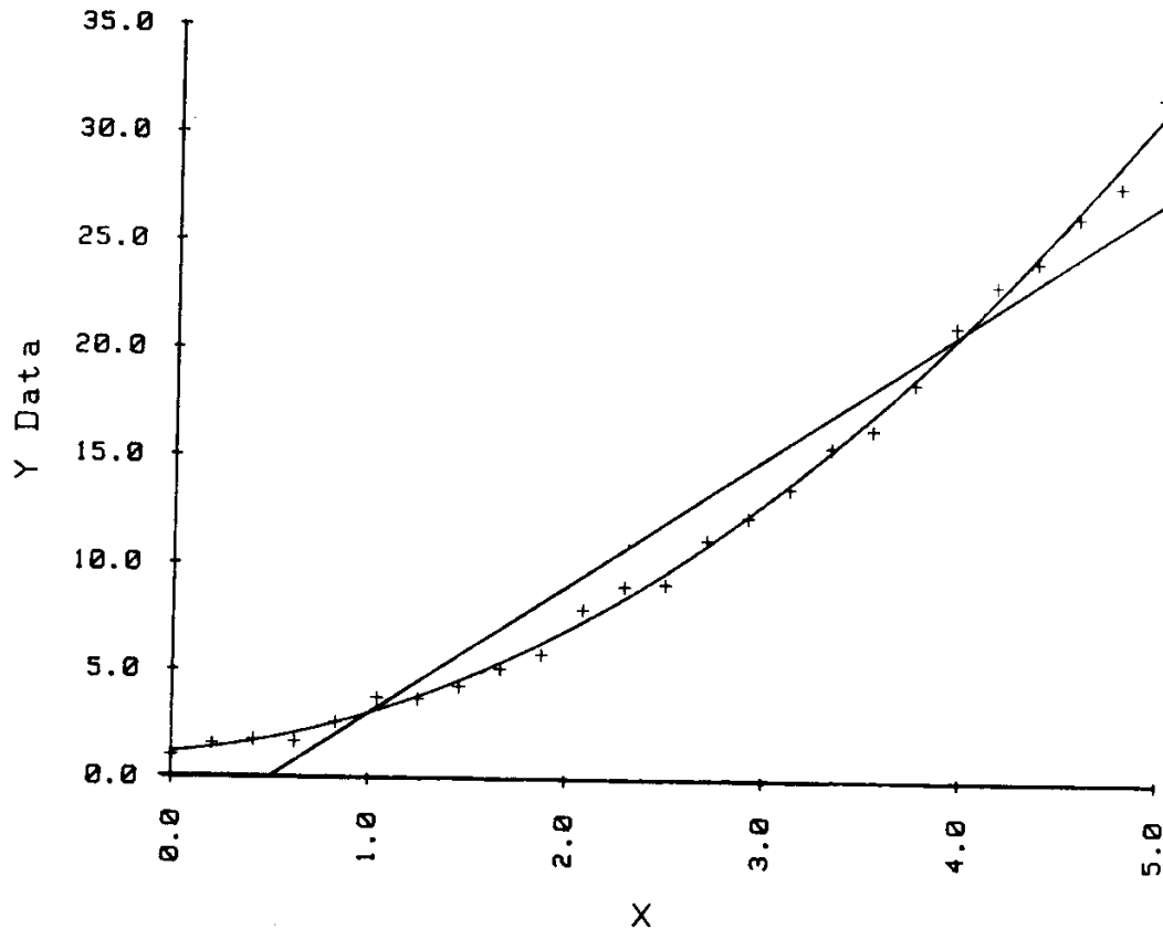
Figura 4-10 Funciones generadas por computadora comparadas con observaciones experimentales.
