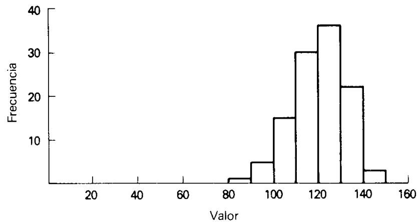
Figura 3-1 Un conjunto de observaciones y su histograma.
