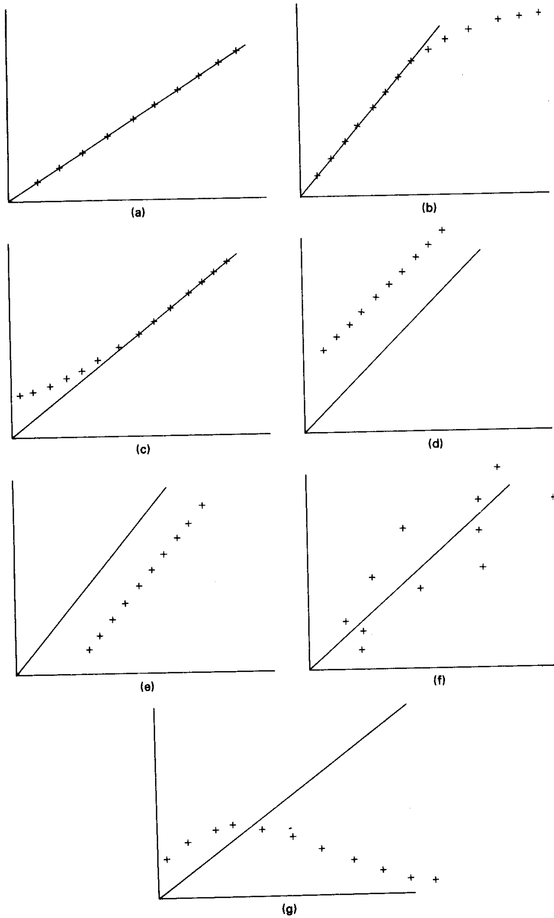
Figura 6-1 La comparación entre sistemas y modelos.
