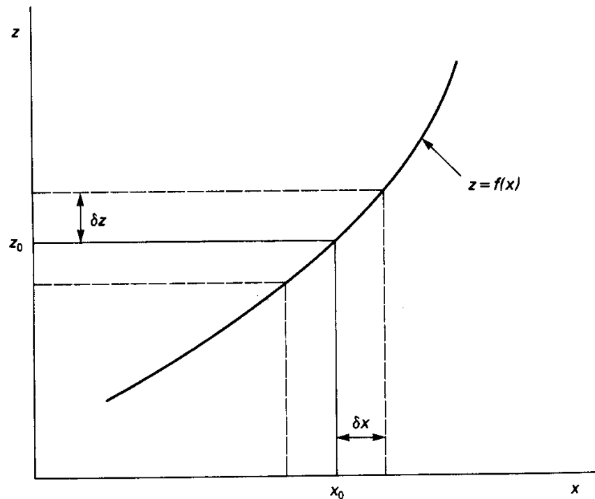
Figura 2-1 Propagación de incertidumbre de una variable a otra.
