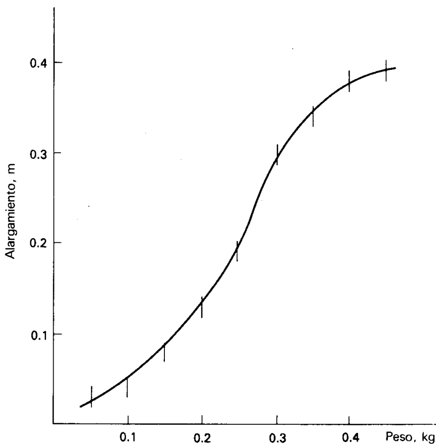
Figura 4-2 Una “curva suave” por las observaciones.
