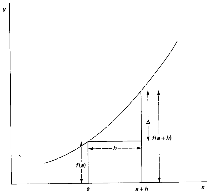
Figura A3-3 Aproximación de la derivada de f(x) en x = a .
