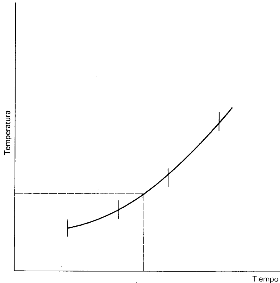
Figura 4-6 Uso potencialmente falaz de la interpolación.
