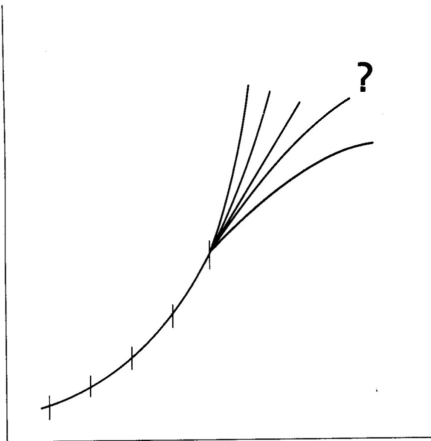
Figura 4-5 La extrapolación no es una de las ciencias exactas.
