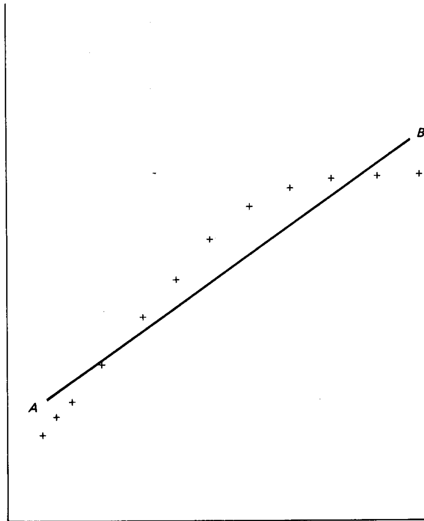
Figura 6-5 Uso inadecuado del ajuste por mínimos cuadrados.
