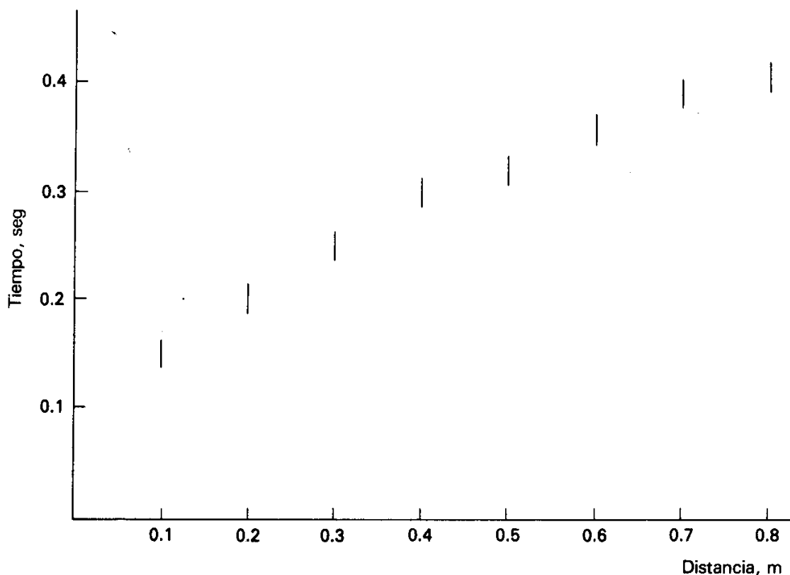
Figura 4-8 Gráfica del tiempo de caída vs. distancia para un objeto con caída libre.
