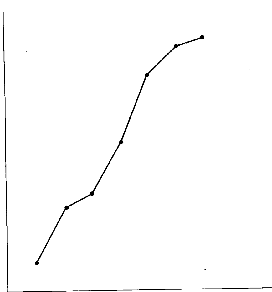
Figura 4-7 Una gráfica que muestra el uso de segmentos lineales.
