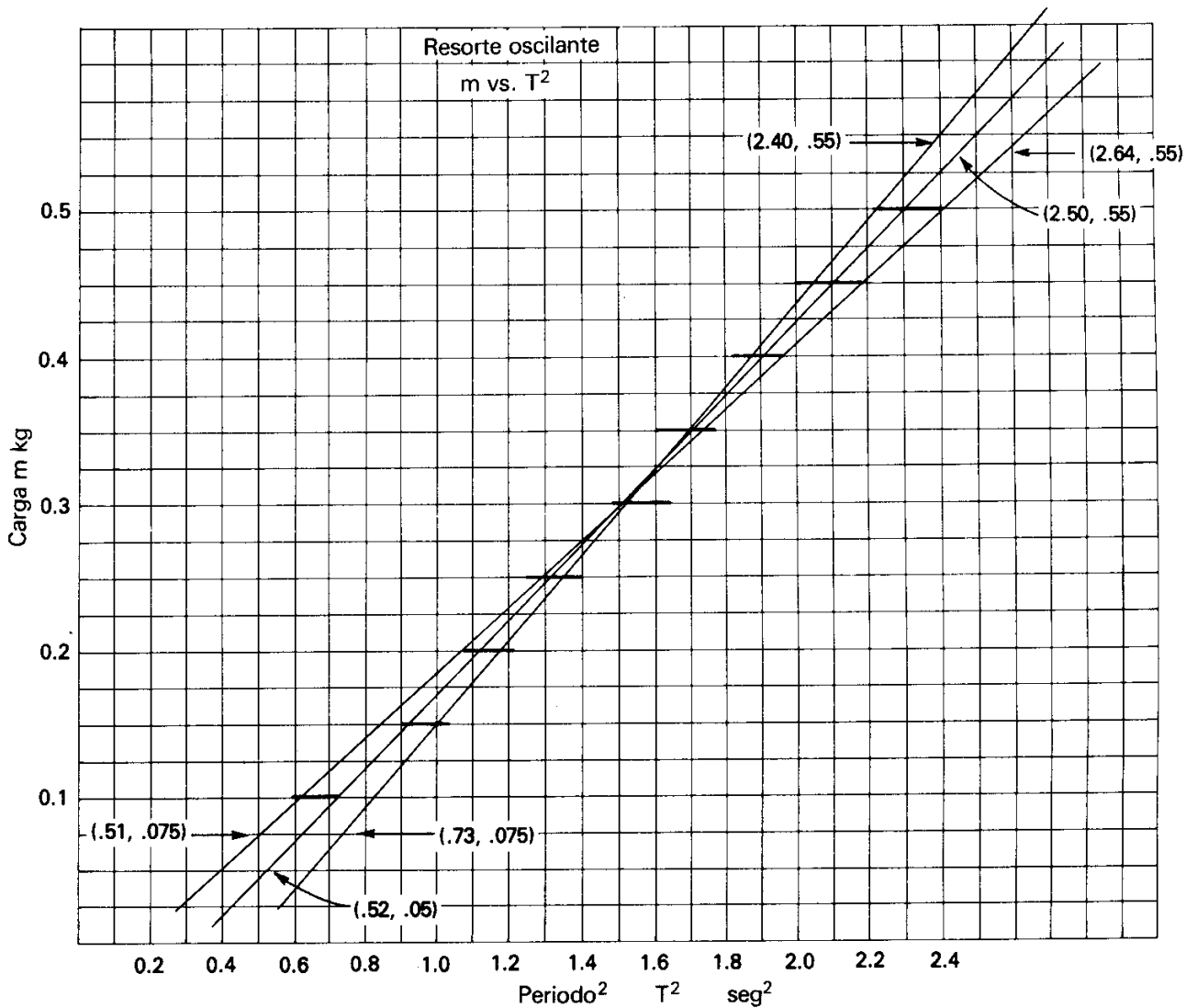
Figura 2 Gráfica de m vs. T^2 .
